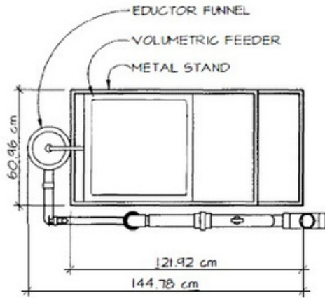
A TOP VIEW SCALE: 1:20
