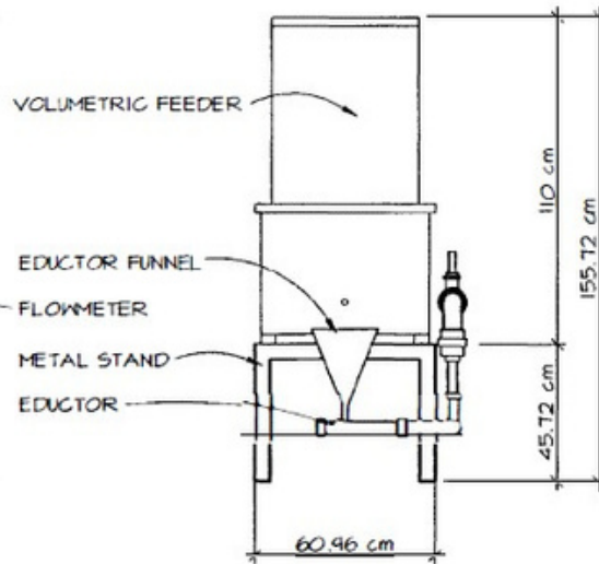
C END VIEW SCALE: 1:20
