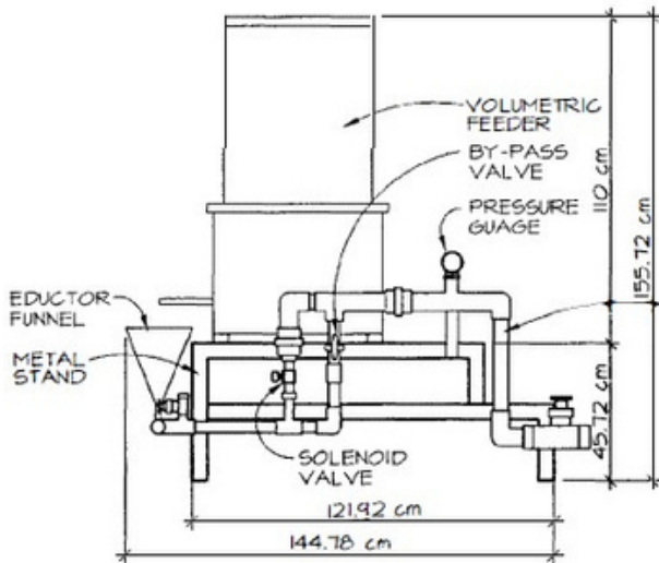
B SIDE VIEW SCALE: 1:20
