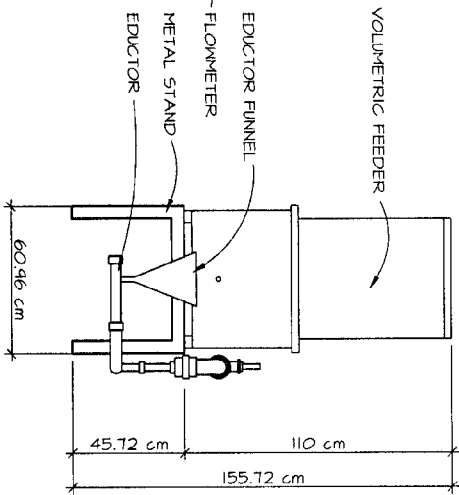
C END VIEW SCALE: 1:20
