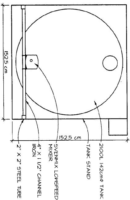
E AGING TANK TOP VIEW SCALE: 1:20
