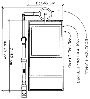
A TOP VIEW SCALE: 1:20
